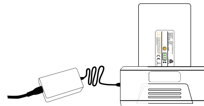
Fig. 9.2.2 Cargado con soporte de carga (accesorio opcional)
