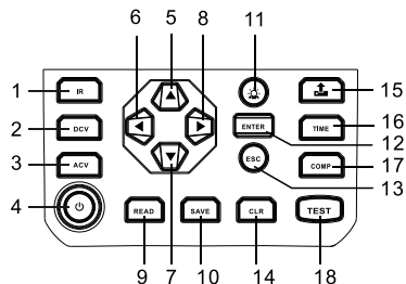
Fig. 6.1 Botones funcionales KRA-2500
