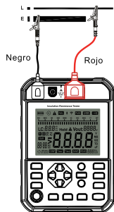
Fig. 9.3.2.1 Conexión por alambre de medición de voltaje
