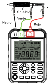
Fig. 10.1.3 Conexión de tres alambres
