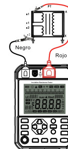
Fig. 10.2.3 Conexión de prueba
