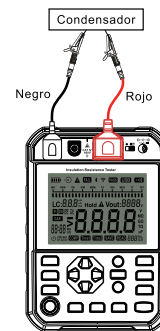
Fig. 9.3.3.1 Conexión de alambre de medición de capacitancia
