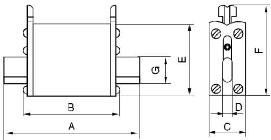
NH00C~NH00
